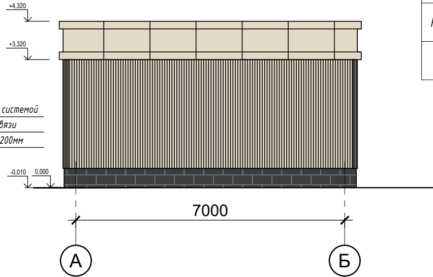
Фасад А-Б
