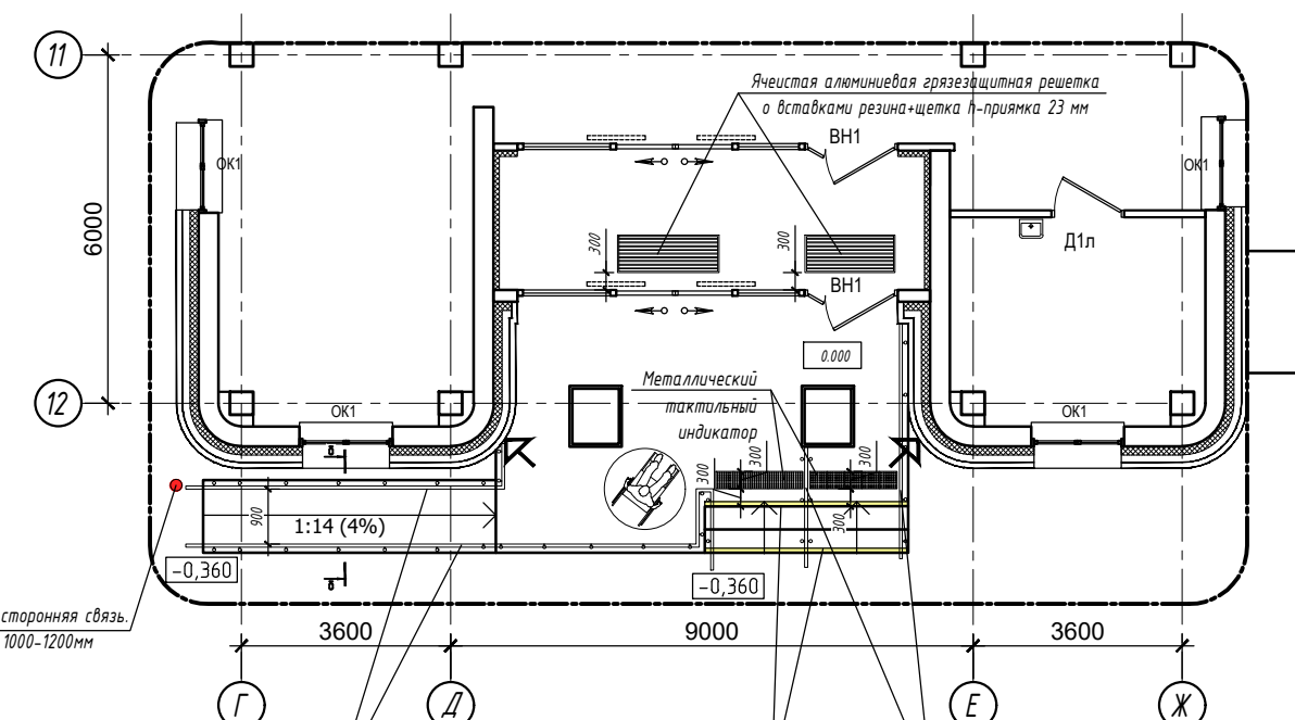
Фрагмент плана
