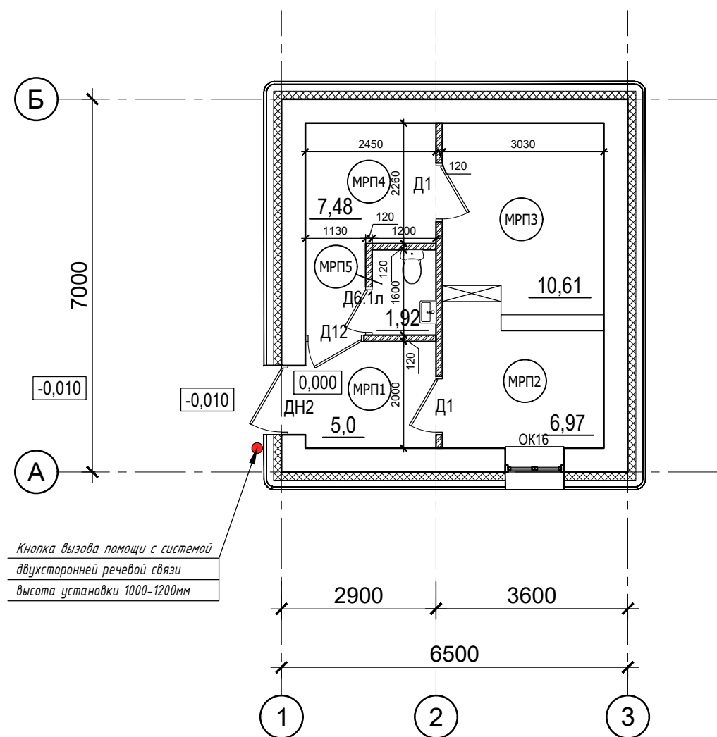
План молочно-раздаточного пункта
