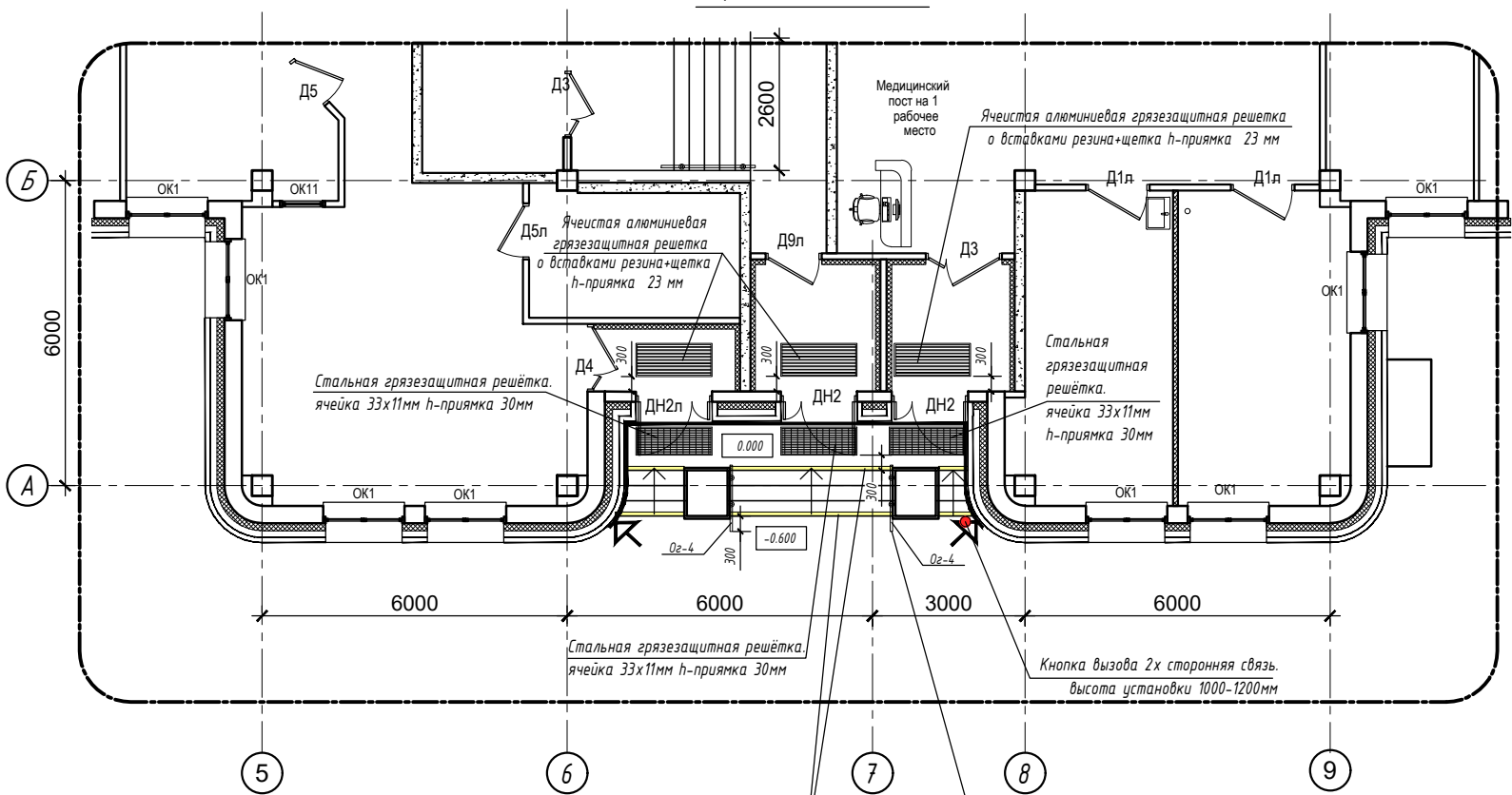
Фрагмент плана
