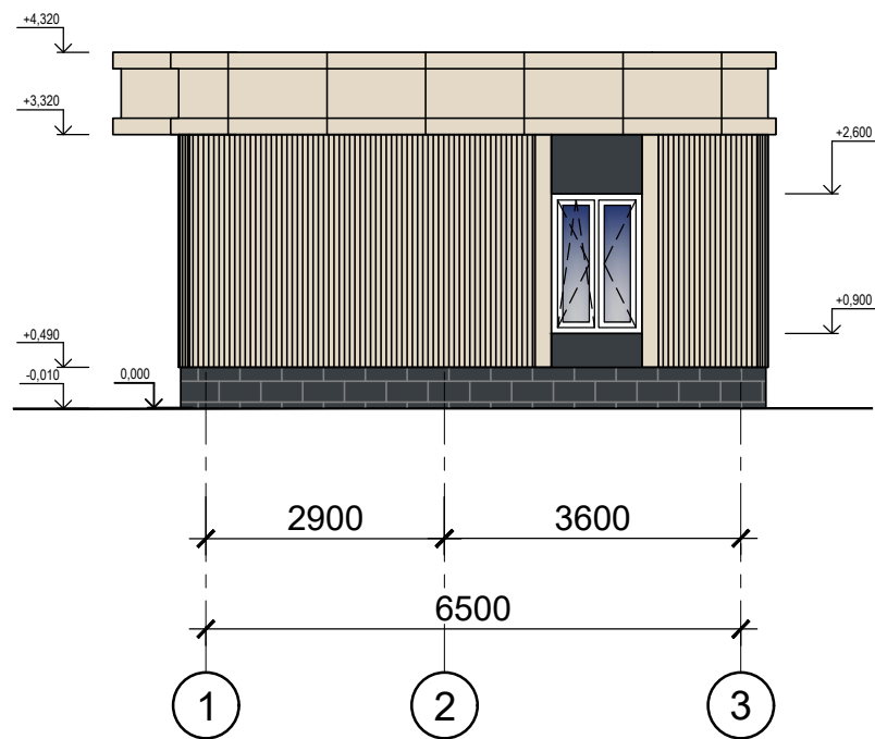
Фасад 1-3
