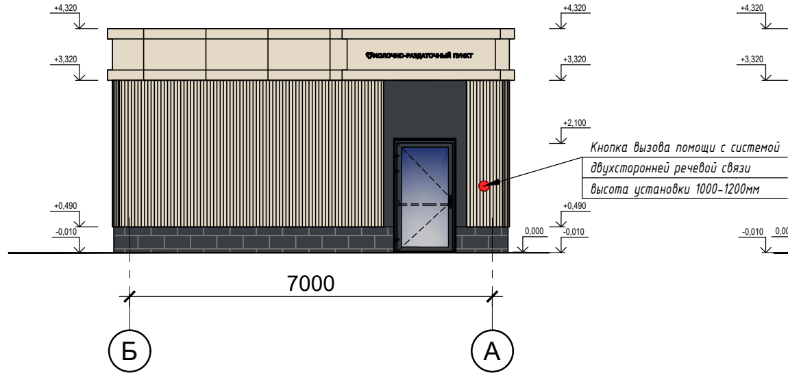
Фасад Б-А
