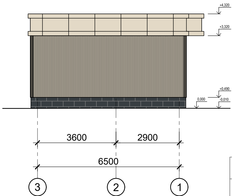
Фасад 3-1
