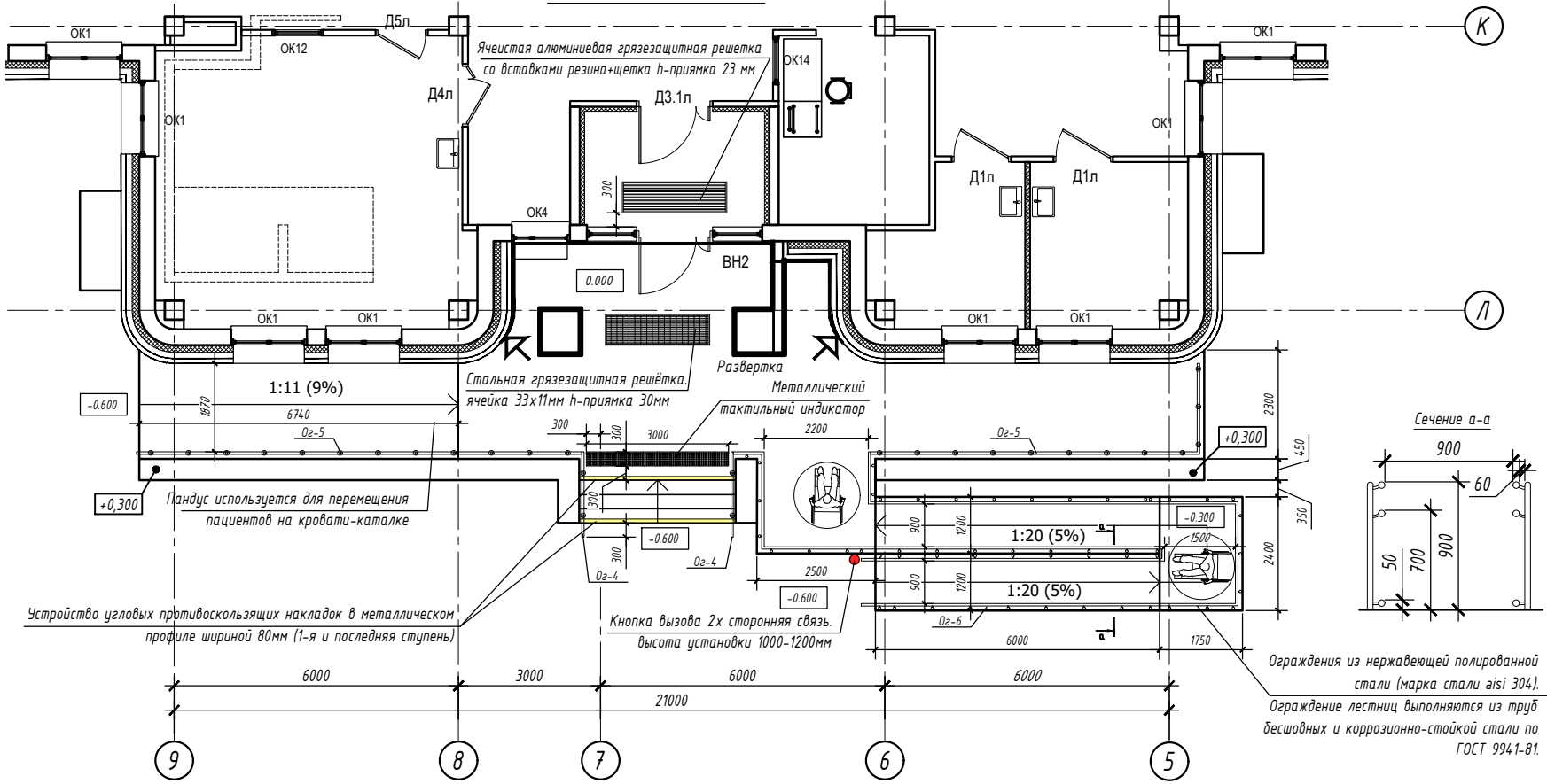
Фрагмент плана
